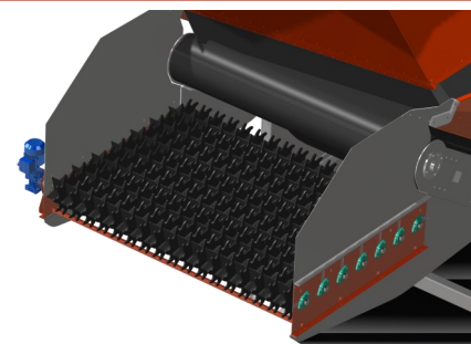
ELIMINADOR DE RAMAS DE ESTRELLAS DIRECTAMENTE EN LA SALIDA DE LA TOLVA (SIN CINTA TRANSVERSAL)
